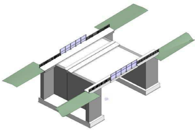
Модель одного из мостов в Autodesk Revit. Изображение предоставлено BPS International.
