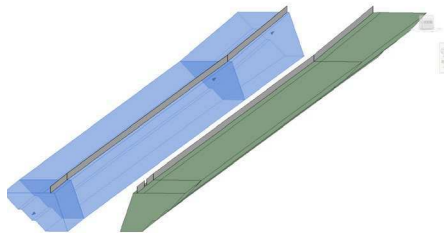
Модель откоса в Autodesk Revit. Изображение предоставлено BPS International.
